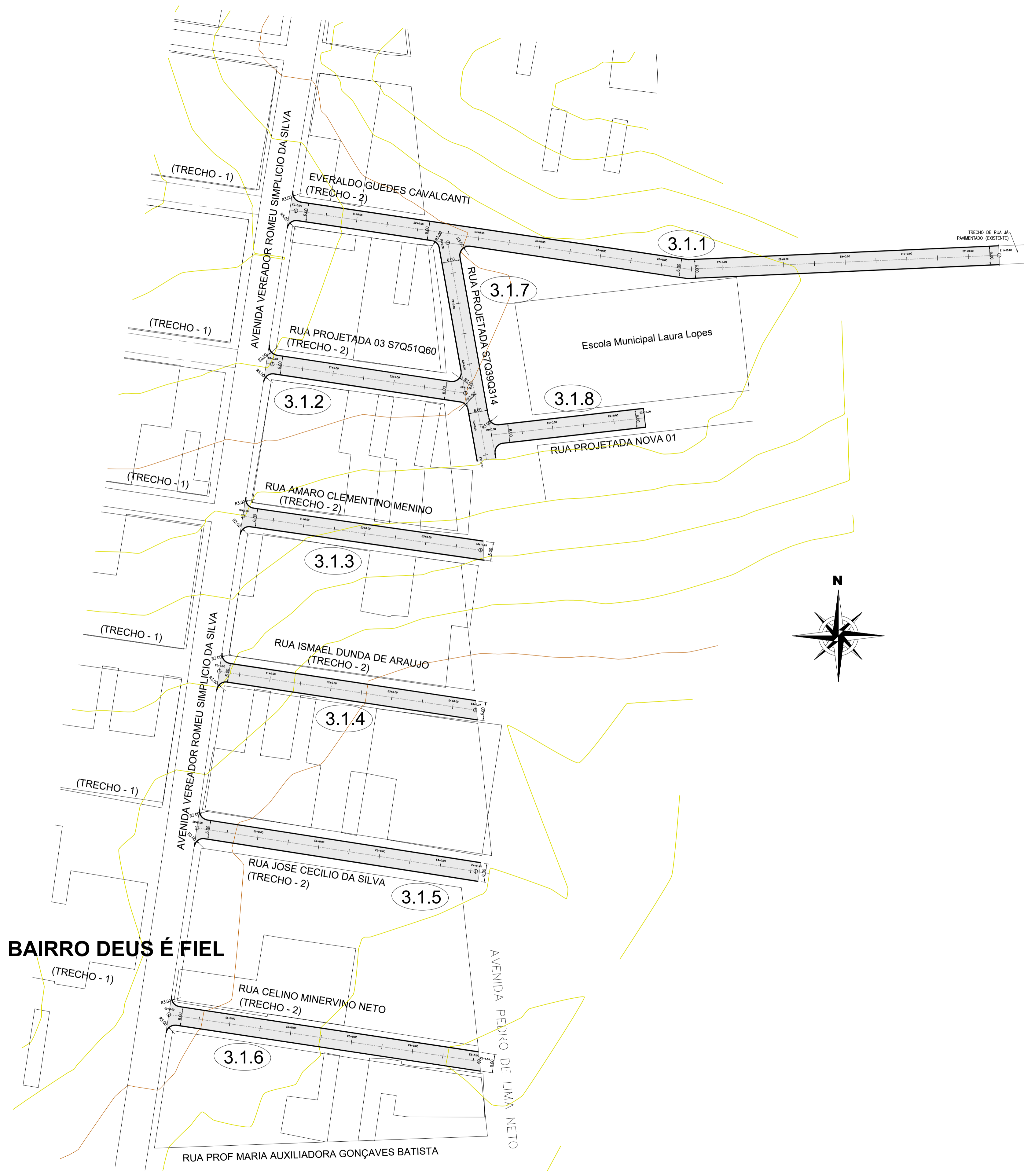
PLANTA DE LOCAÇÃO - GERAL ESCALA: 1/750
