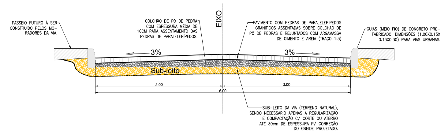
SEÇÃO TRANSVERSAL (Tipo) SEM ESCALA
