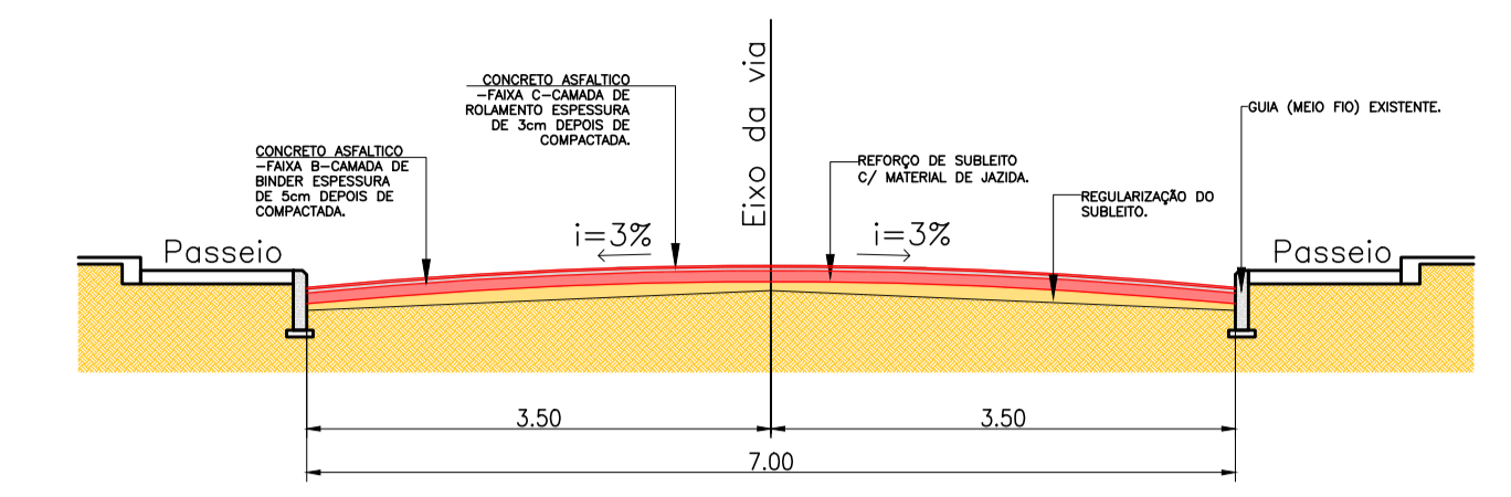
SEÇÃO TIPO SEM ESCALA
