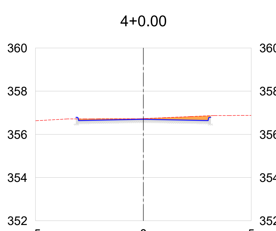
SEÇÕES TRANSVERSAIS - RUA FRANCISCO COELHO DE LIMA 2 Escala: H = 1 / 1000 V = 1 / 100
