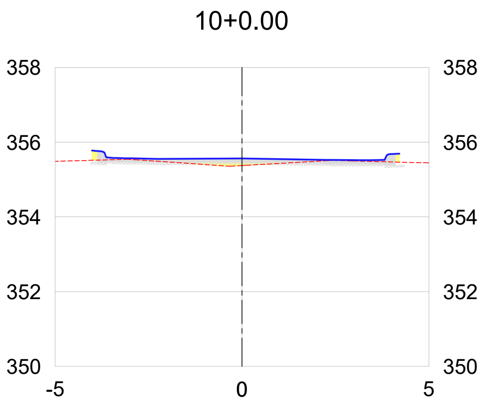
SEÇÕES TRANSVERSAIS - OTAVIANO FLORIANO DA SILVA 1 Escala: H = 1 / 1000 V = 1 / 100
