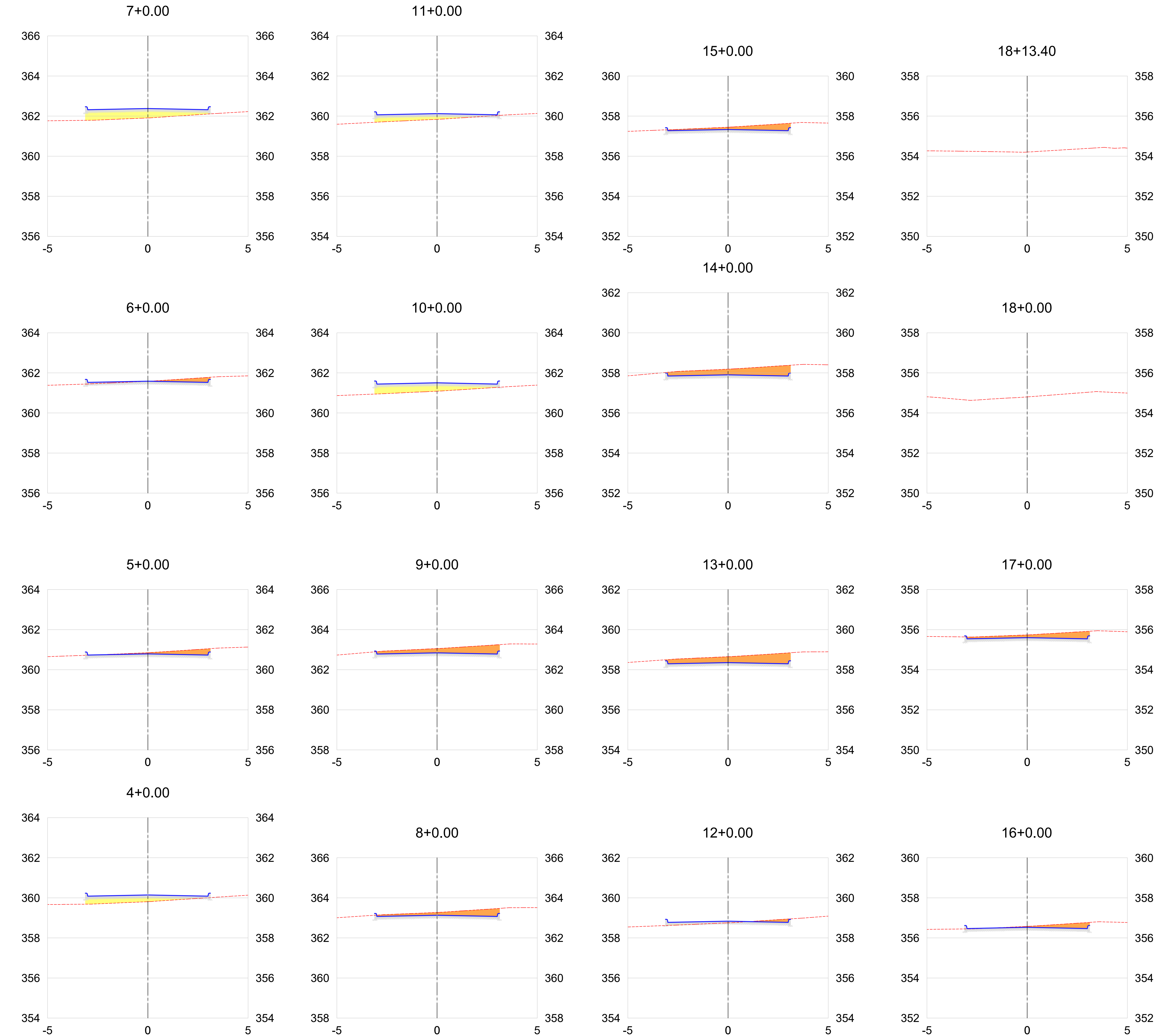
1 SEÇÕES TRANSVERSAIS - RUA FRANCISCO DAS CHAGAS DE LIMA
