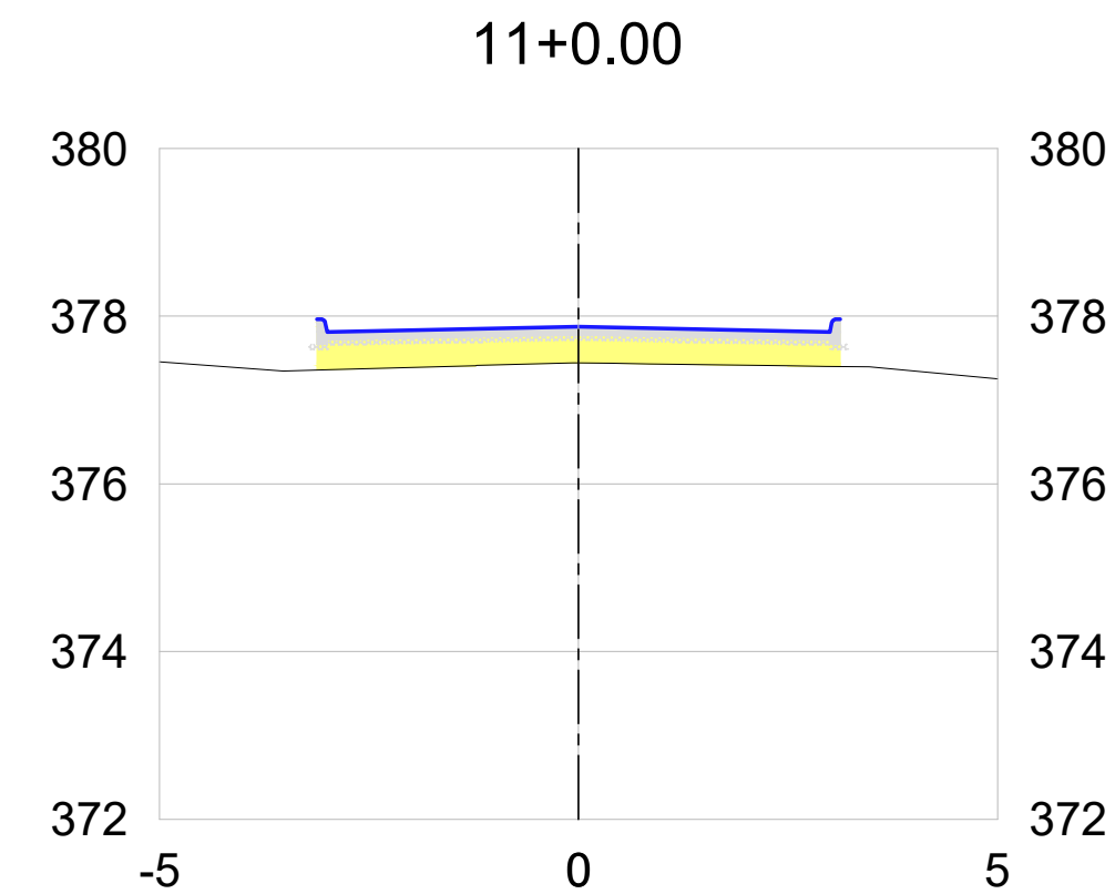
1 SEÇÕES TRANSVERSAIS - RUA LAURA LOPES TAVARES DA SILVA
