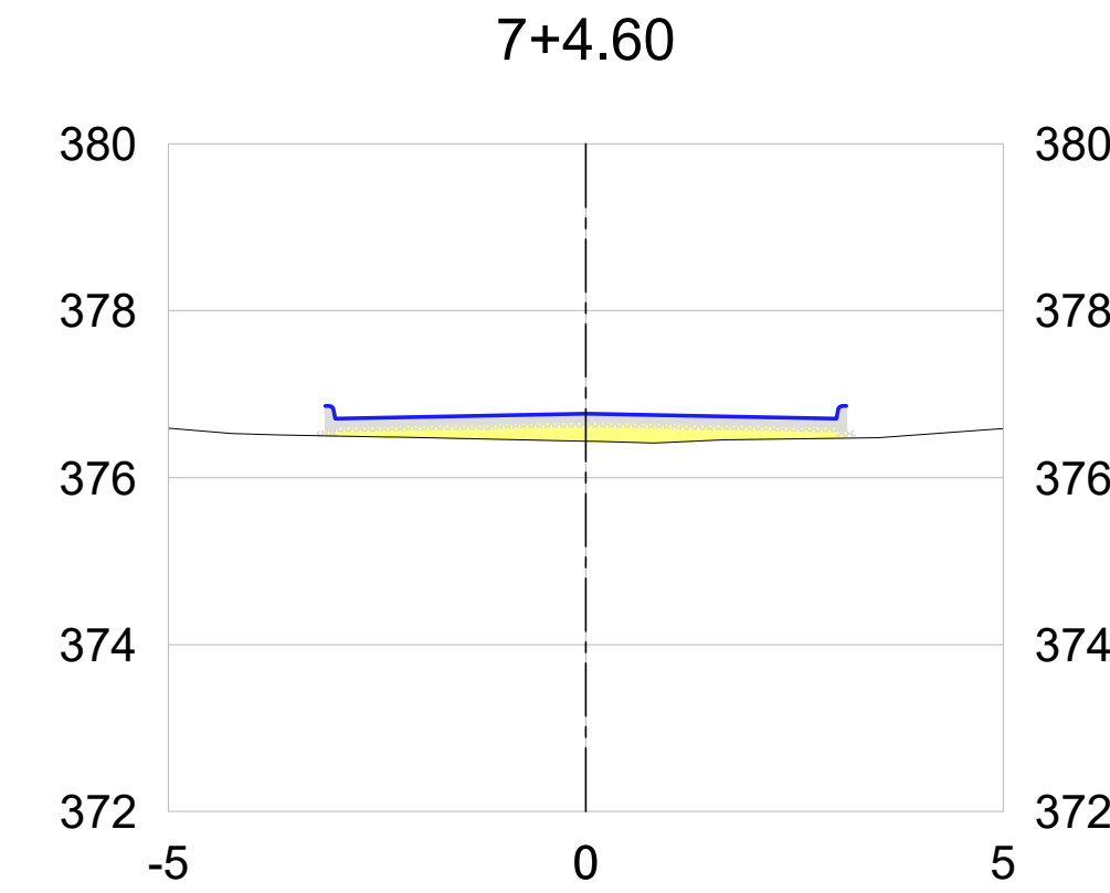
3 SEÇÕES TRANSVERSAIS - RUA PROJETADA "X"
