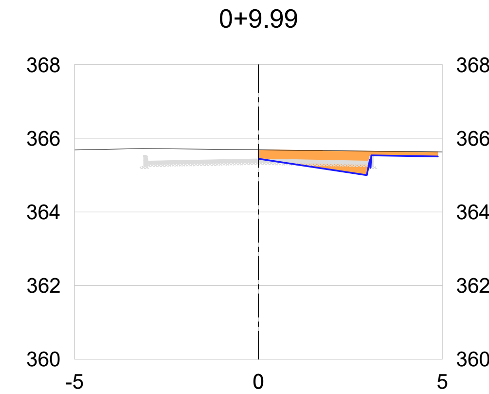
2 SEÇÕES TRANSVERSAIS - RUA PROJETADA "X"
