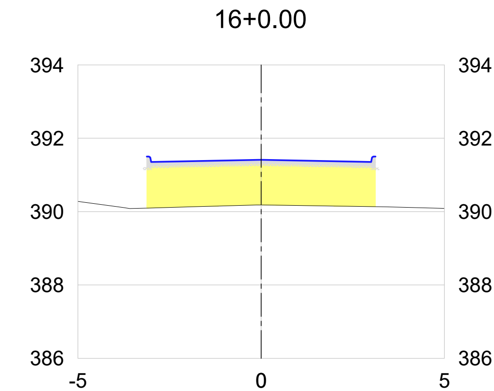
1 SEÇÕES TRANSVERSAIS - RUA LAURA LOPES TAVARES DA SILVA
