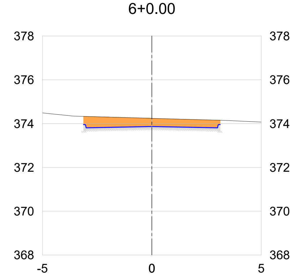
3 SEÇÕES TRANSVERSAIS - RUA PROJETADA "X"
