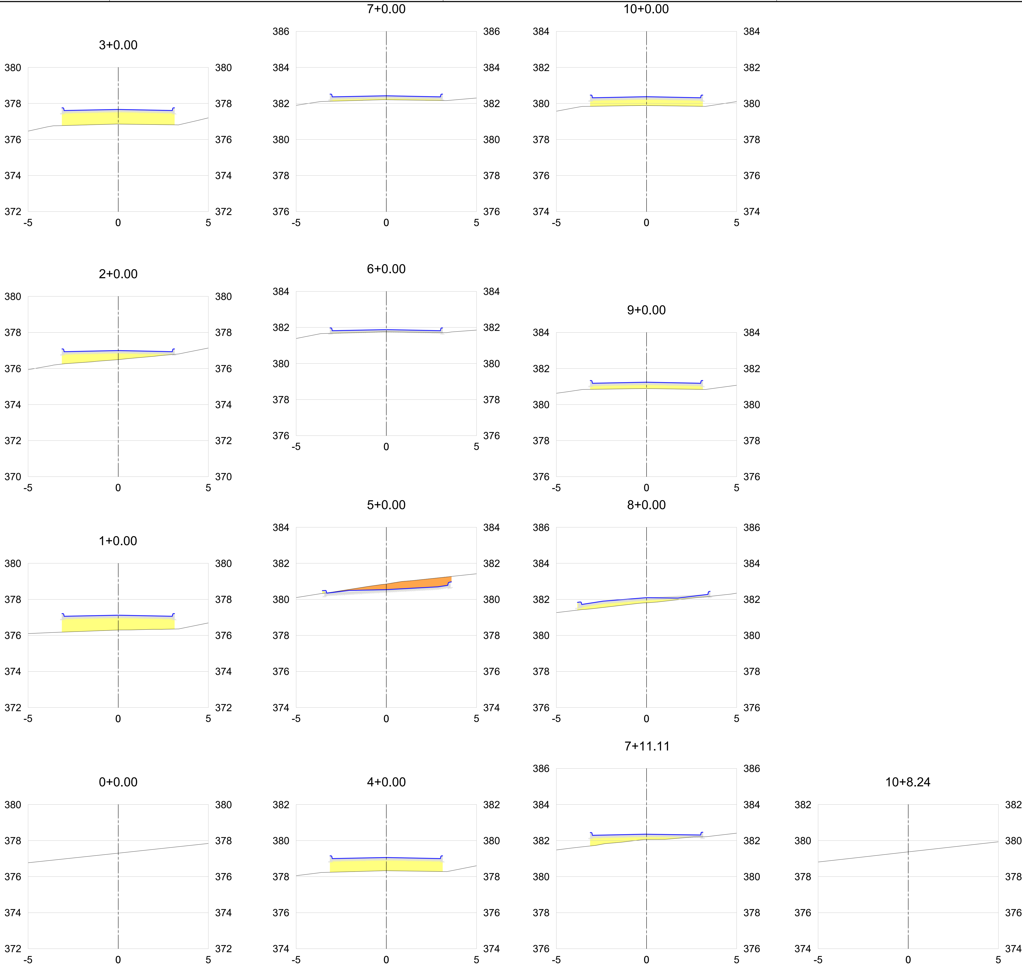
1 SEÇÕES TRANSVERSAIS - RUA DIEGO ARTHUR DA SILVA Escala: H = 1 / 1000 V = 1 / 100
