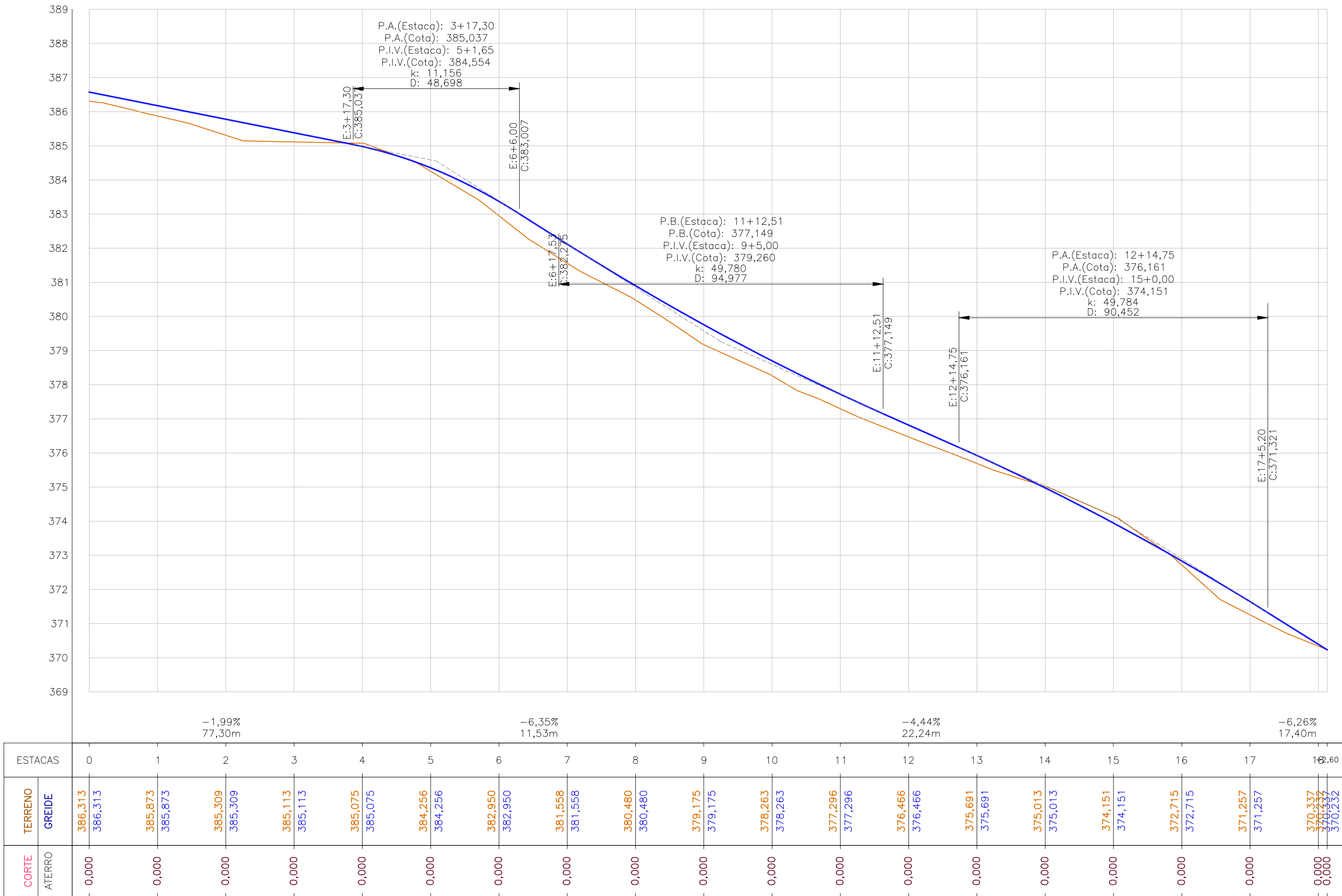
2 PERFIL LONGITUDINAL Escala: H = 1 / 1000 V = 1 / 100
