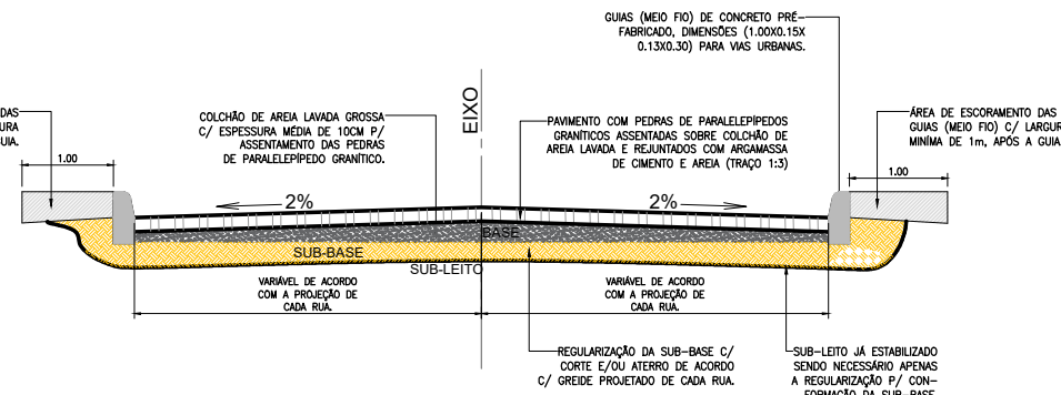
4 SEÇÃO TIPO PROJETADA Sem escala
