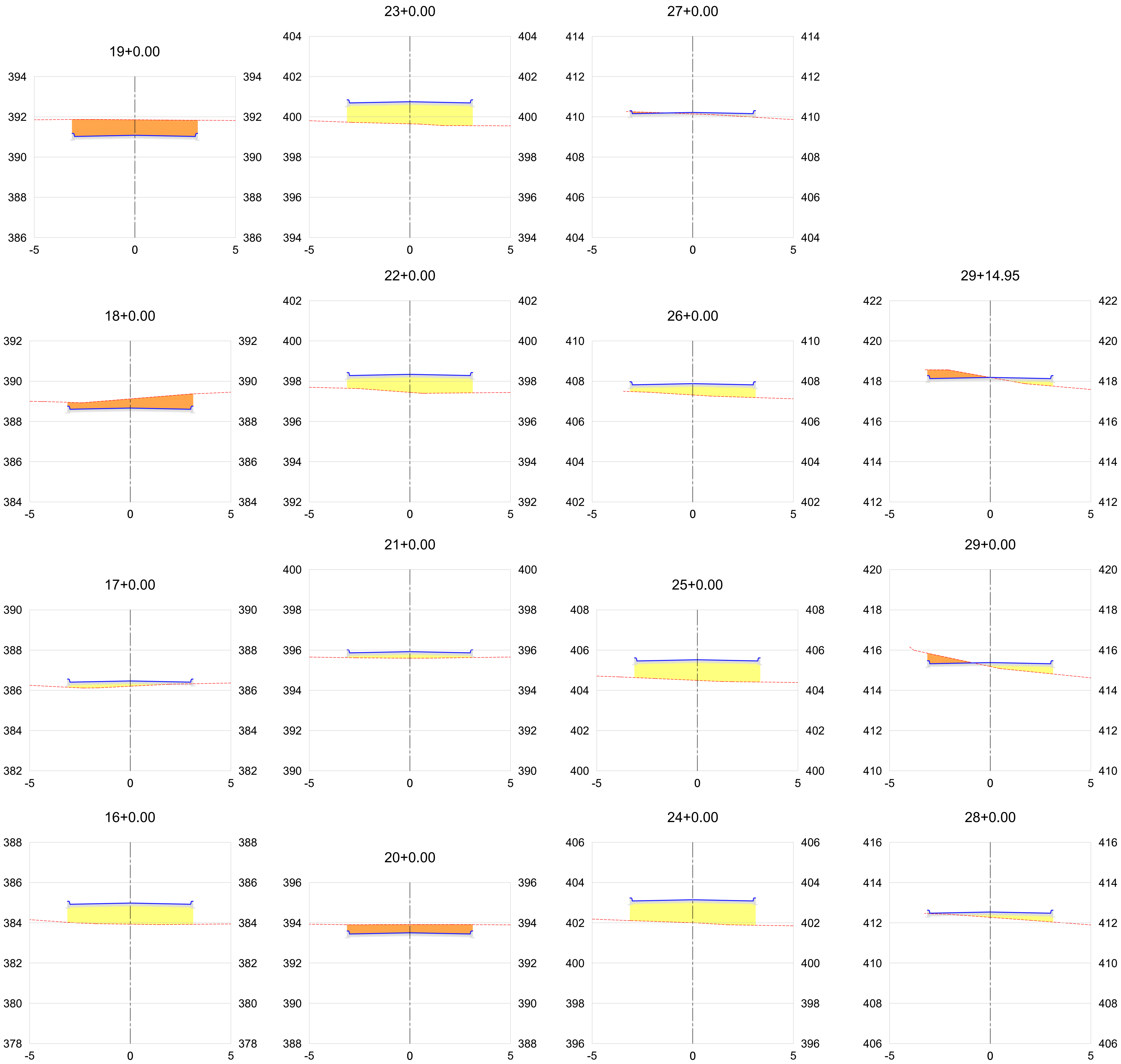
1 SEÇÕES TRANSVERSAIS - RUA EDITE LURDES DA SILVA Escala: H = 1 / 1000 V = 1 / 100
