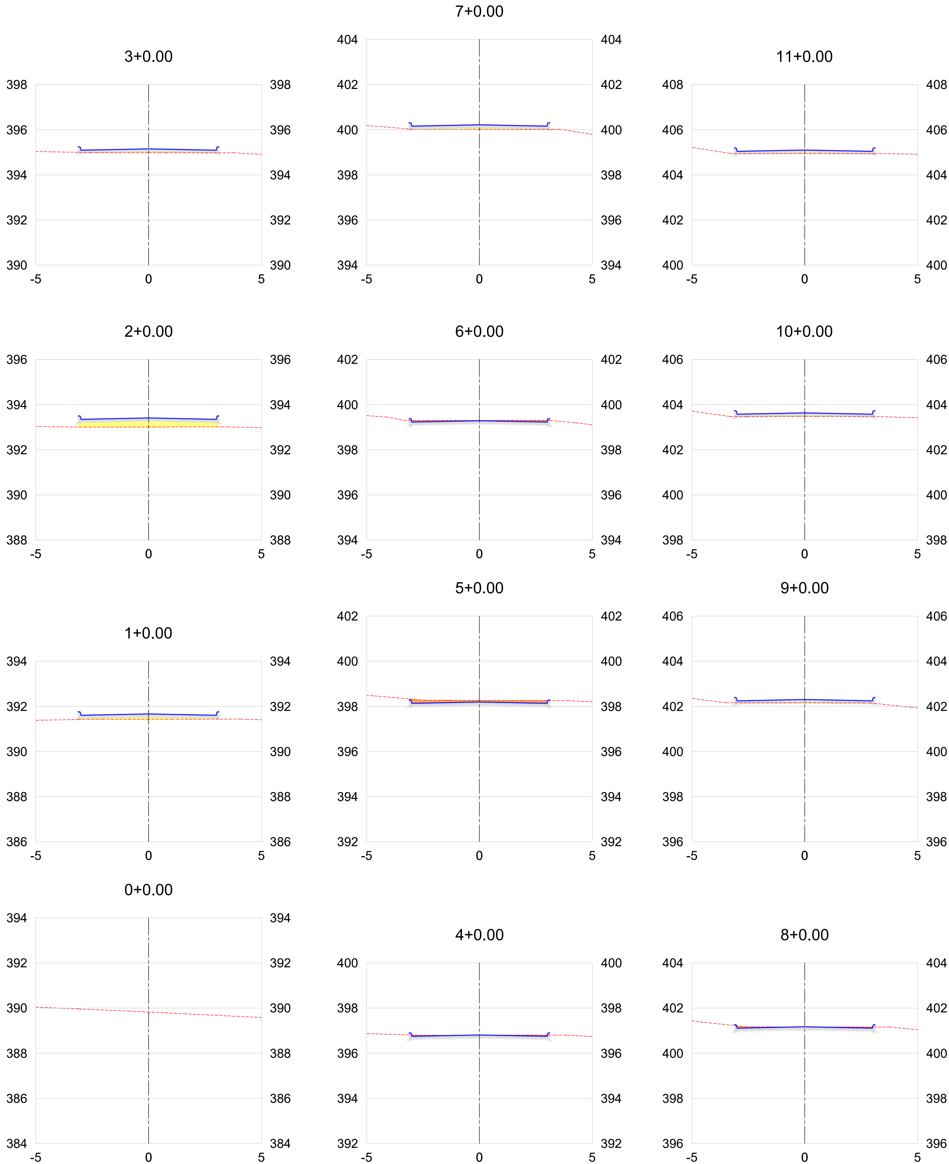
1 SEÇÕES TRANSVERSAIS - RUA VEREADOR LUIS GALDINO Escala: H = 1 / 1000 V = 1 / 100
