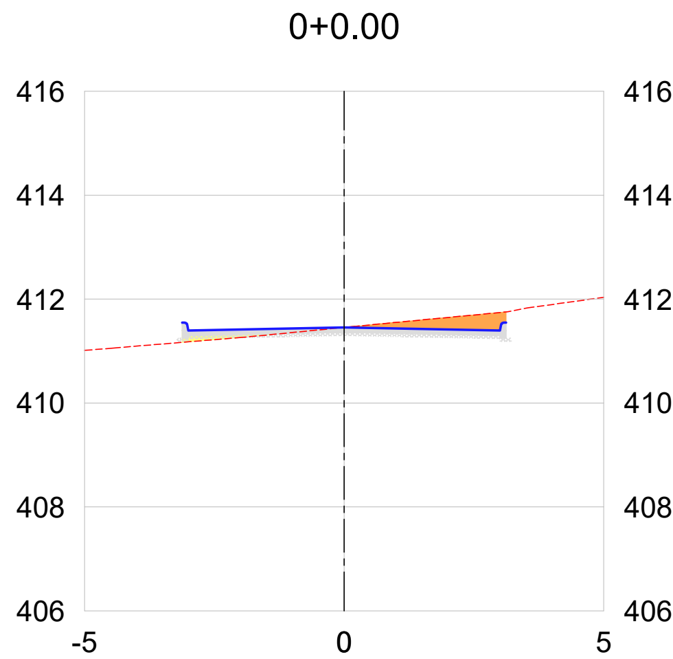
2 SEÇÕES TRANSVERSAIS - RUA JOSE ALFREDO DA SILVA - Trecho 1 Escala: H = 1 / 1000 V = 1 / 100
