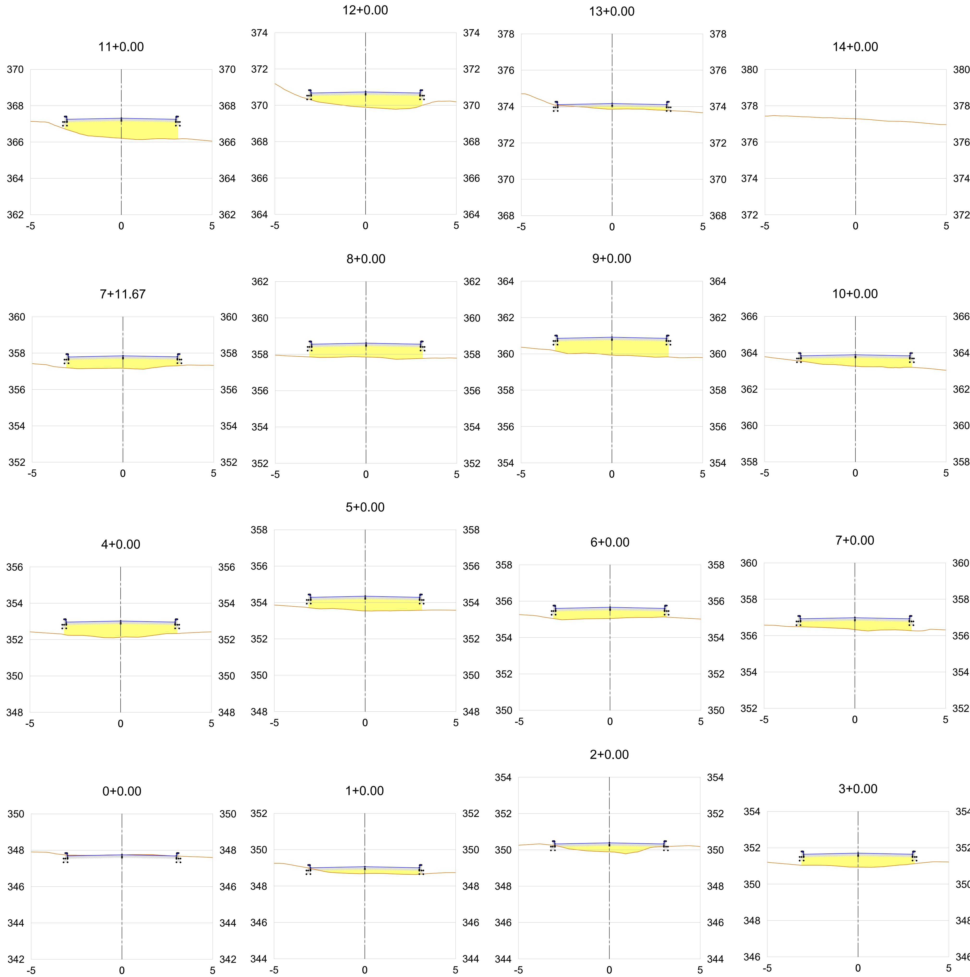
1 SEÇÕES TRANSVERSAIS - RUA JOSÉ MIGUEL Escala: H = 1 / 1000 V = 1 / 100
