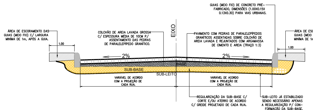
2 SEÇÃO TIPO PROJETADA Sem escala
