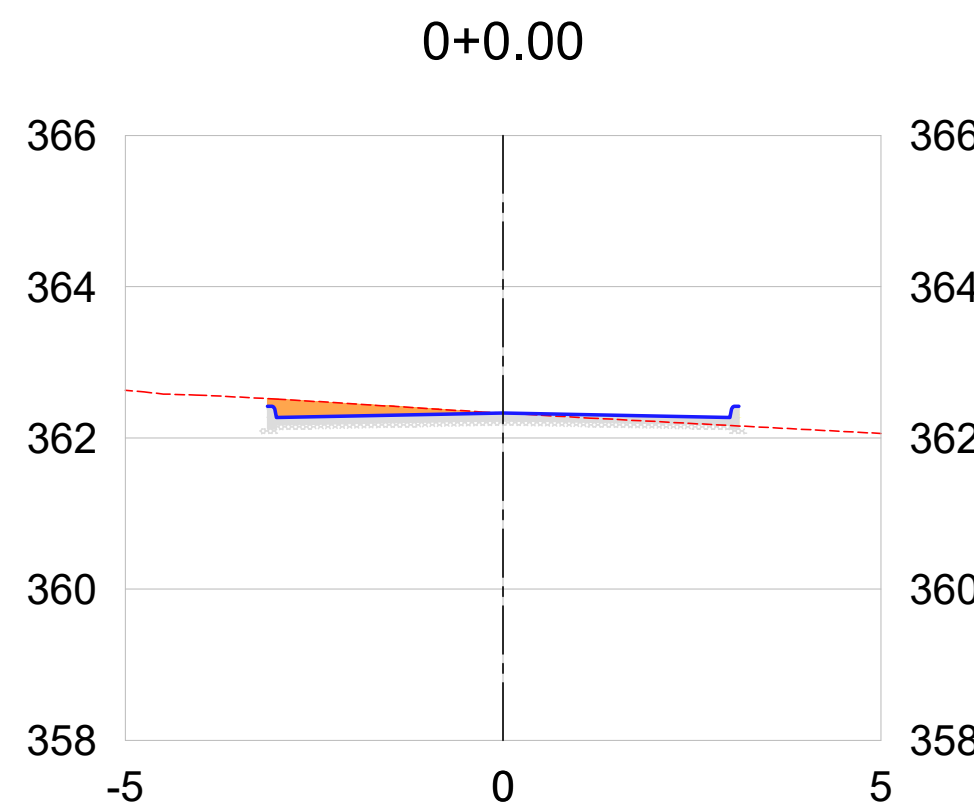
SEÇÕES TRANSVERSAIS - RUA OSCAR FERREIRA DA SILVA
