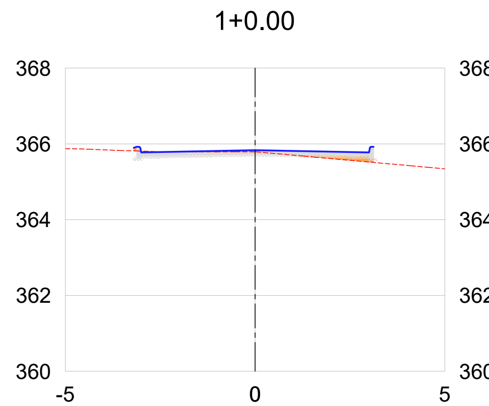
SEÇÕES TRANSVERSAIS - RUA LUZINETE ELIAS DE LIMA
