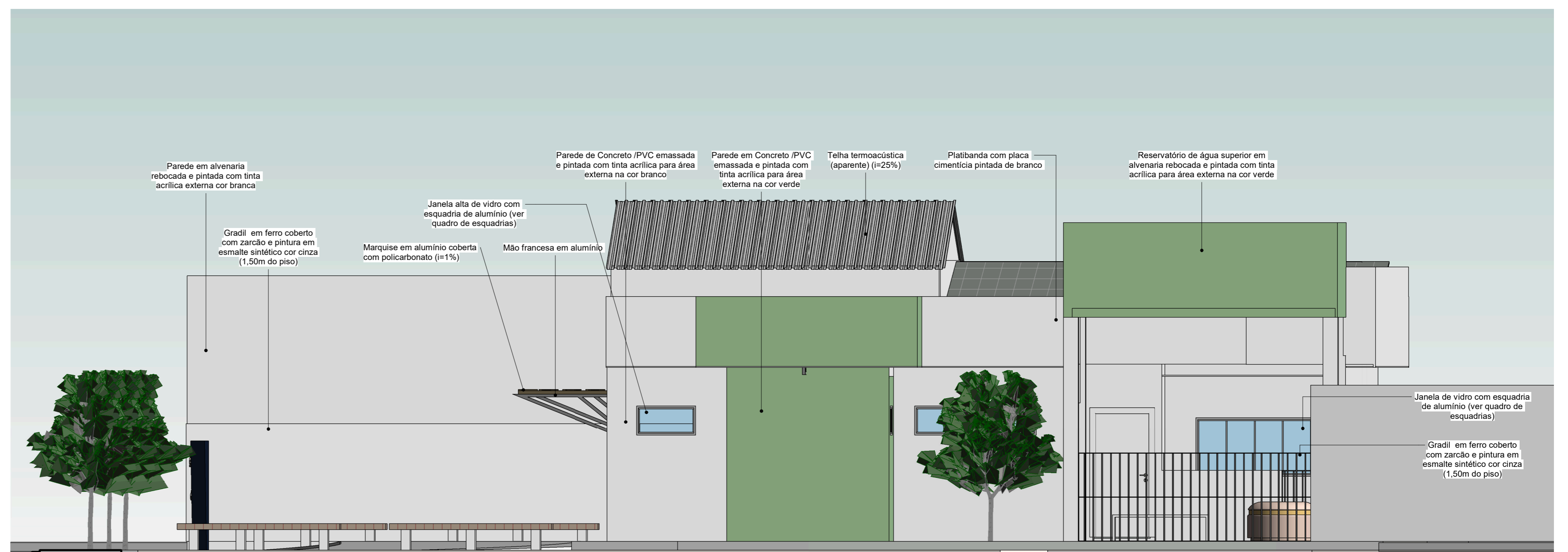
4 FACHADA OESTE ESCALA 1:50
