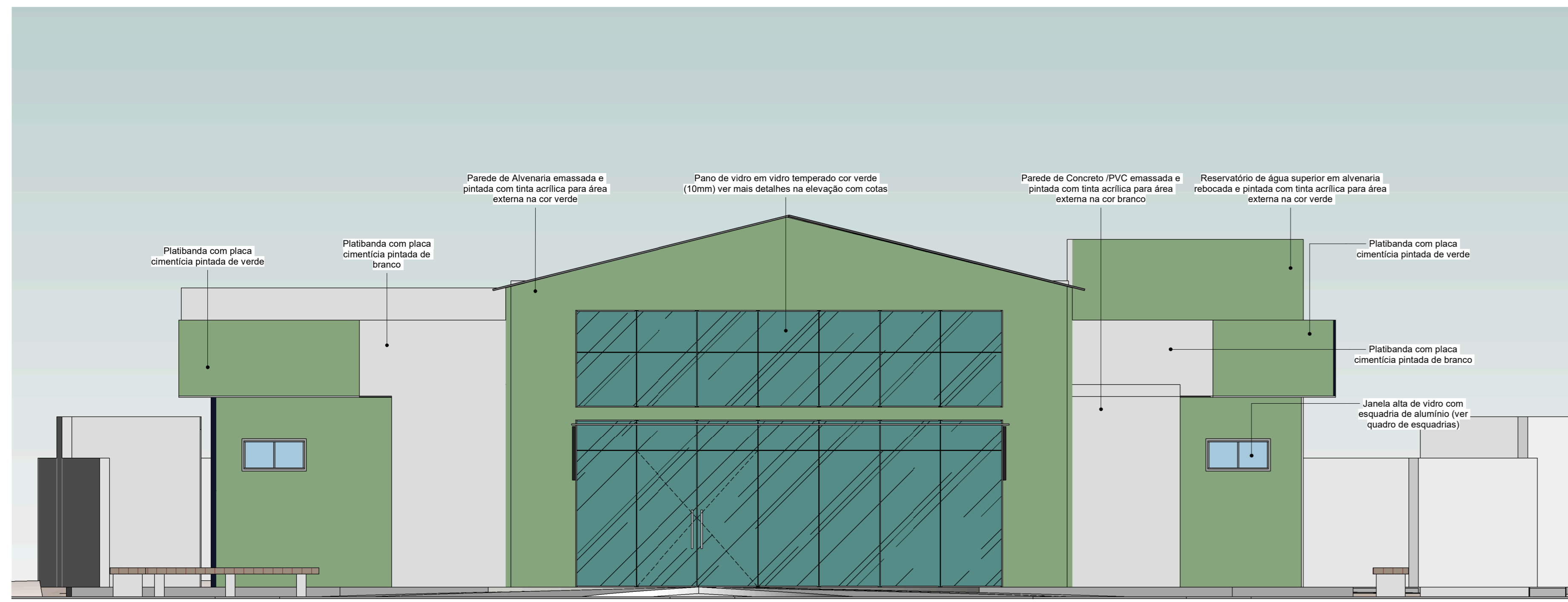
1 FACHADA NORTE ESCALA 1:50
